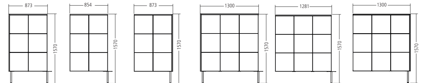
4813-084 module 2 x 3
