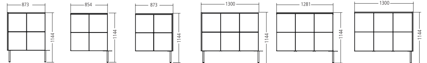
4812-084 module 2 x 2
