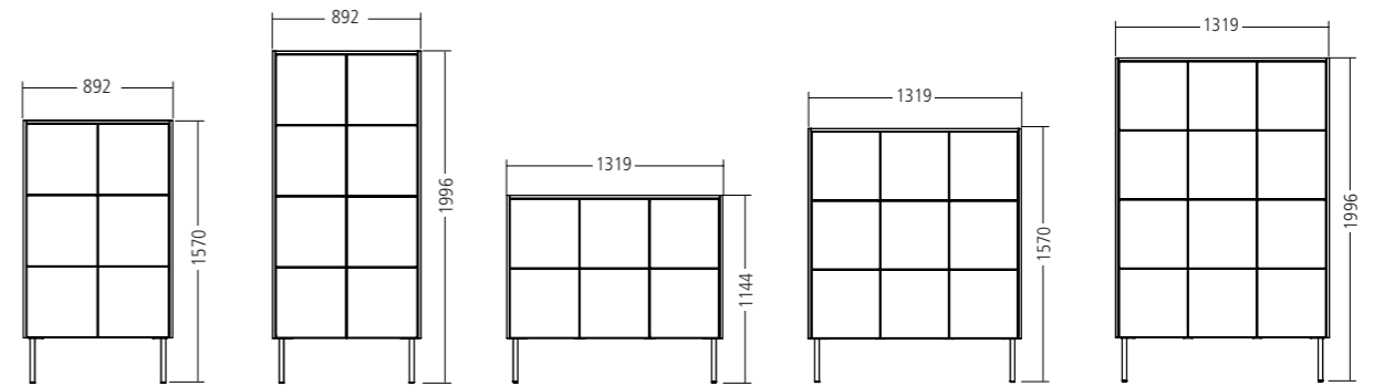
4803-084 Locker 2 x 3
