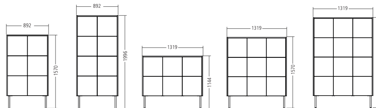
4803-084 Armoire 2 x 3 4804-084 Armoire 2 x 4 4802-124 Armoire 3 x 2 4803-124 Armoire 3 x 3 4804-124 Armoire 3 x 4
