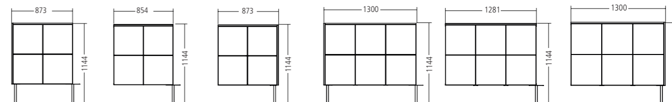
4812-084 module 2 x 2 panneau extérieur, côté gauche 4822-084 module 2 x 2 module central 4832-084 module 2 x 2 panneau extérieur, côté droit 4812-124 module 3 x 2 panneau extérieur, côté gauche 4822-124 module 3 x 2 module central 4832-124 module 3 x 2 panneau extérieur, côté droit
