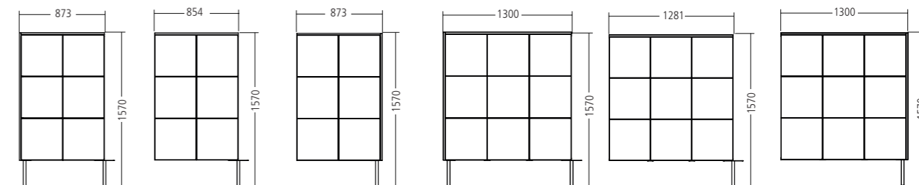
4813-084 module 2 x 3 panneau extérieur, côté gauche 4823-084 module 2 x 3 module central 4833-084 module 2 x 3 panneau extérieur, côté droit 4813-124 module 3 x 3 panneau extérieur, côté gauche 4823-124 module 3 x 3 module central 4833-124 module 3 x 3 panneau extérieur, côté droit
