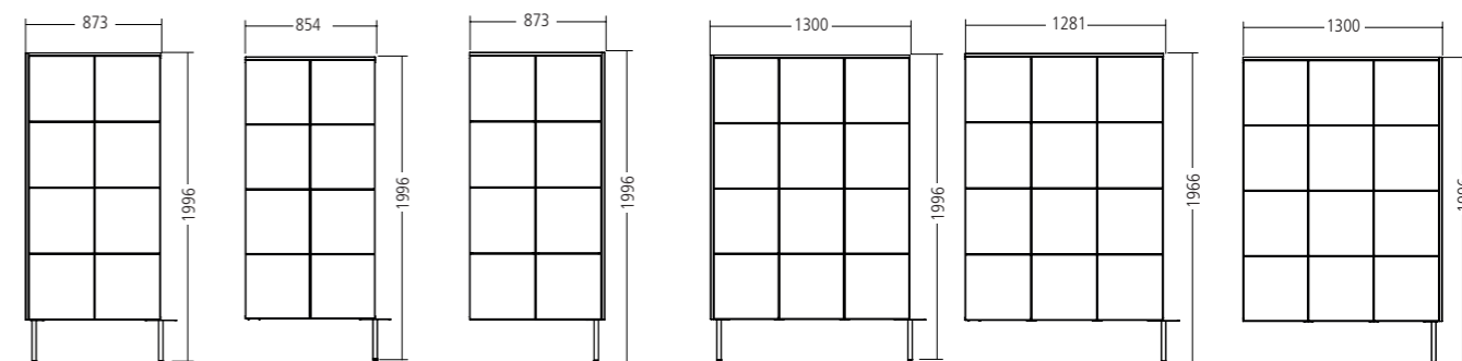
4814-084 Modul 2 x 4 panneau extérieur, côté gauche 4824-084 Modul 2 x 4 module central 4834-084 Modul 2 x 4 panneau extérieur, côté droit 4814-124 Modul 3 x 4 panneau extérieur, côté gauche 4824-124 Modul 3 x 4 module central 4834-124 Modul 3 x 4 panneau extérieur, côté droit
