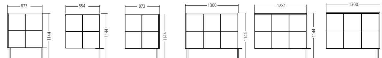
4812-084 modul 2 x 2 krycí deska vlevo 4822-084 modul 2 x 2 střed 4832-084 modul 2 x 2 krycí deska vpravo 4812-124 modul 3 x 2 krycí deska vlevo 4822-124 modul 3 x 2 střed 4832-124 modul 3 x 2 krycí deska vpravo
