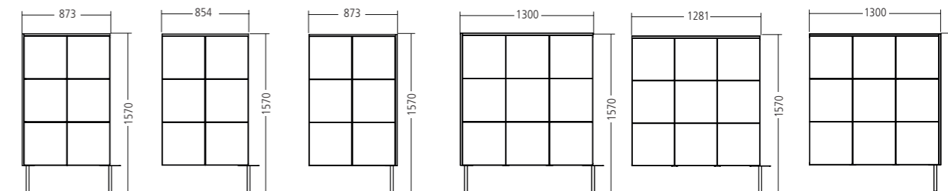
4813-084 modul 2 x 3 krycí deska vlevo 4823-084 modul 2 x 3 střed 4833-084 modul 2 x 3 krycí deska vpravo 4813-124 modul 3 x 3 krycí deska vlevo 4823-124 modul 3 x 3 střed 4833-124 modul 3 x 3 krycí deska vpravo
