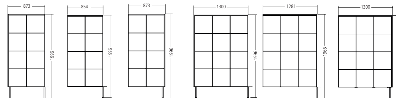
4814-084 modul 2 x 4 krycí deska vlevo 4824-084 modul 2 x 4 střed 4834-084 modul 2 x 4 krycí deska vpravo 4814-124 modul 3 x 4 krycí deska vlevo 4824-124 modul 3 x 4 střed 4834-124 modul 3 x 4 krycí deska vpravo
