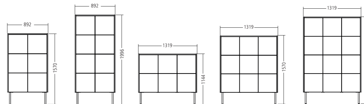
4803-084 Skříň 2 x 3 4804-084 Skříň 2 x 4 4802-124 Skříň 3 x 2 4803-124 Skříň 3 x 3 4804-124 Skříň 3 x 4
