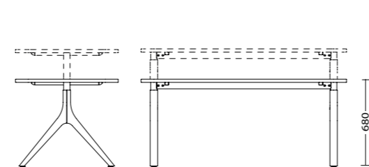
Tafelhoogte manueel verstelbaar
